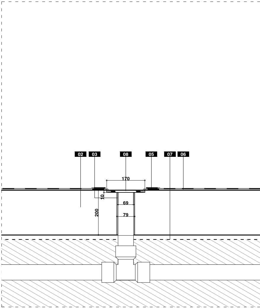
Detalle 2
